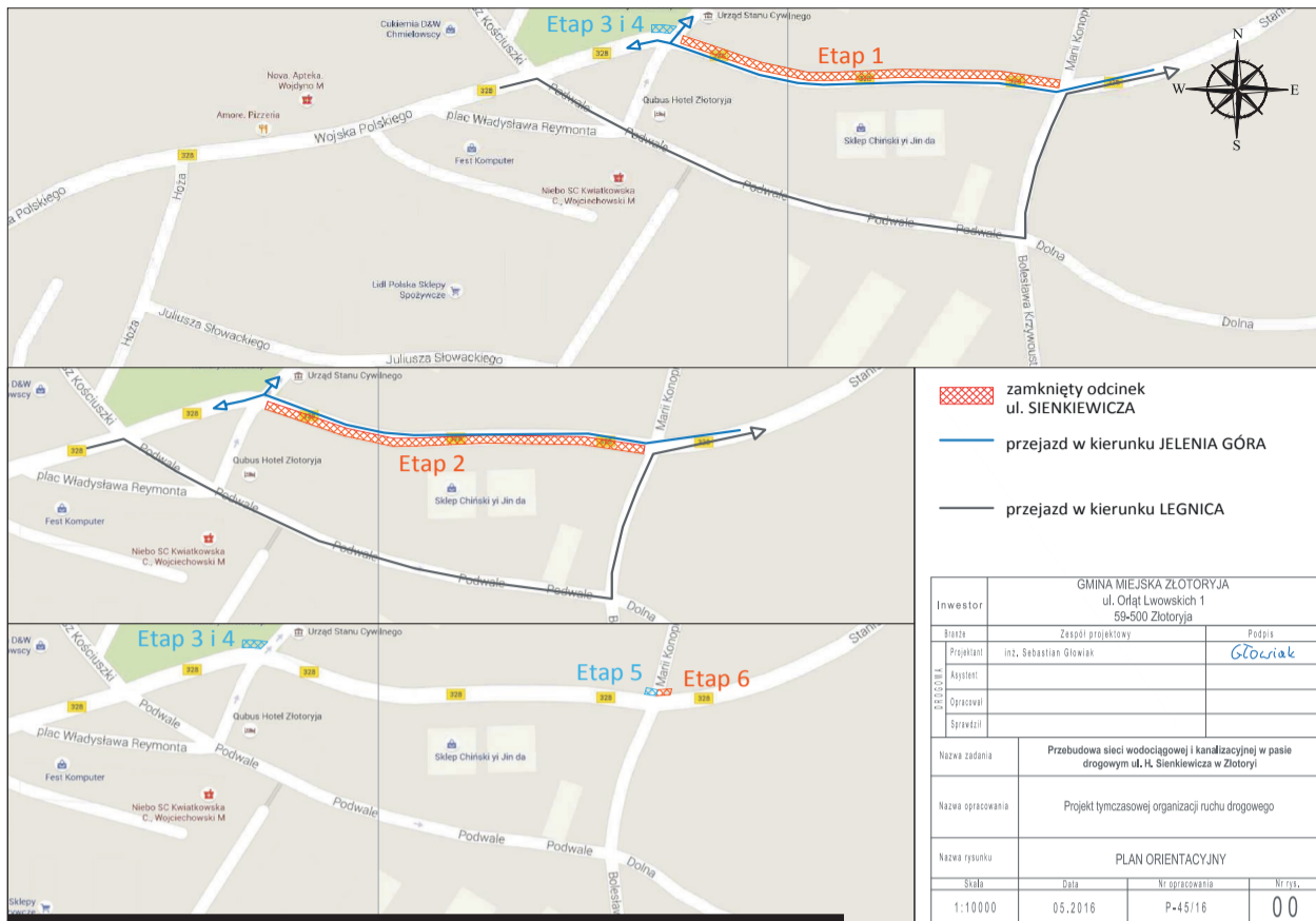
Schemat objazdów podczas remontu ul. Sienkiewicza
